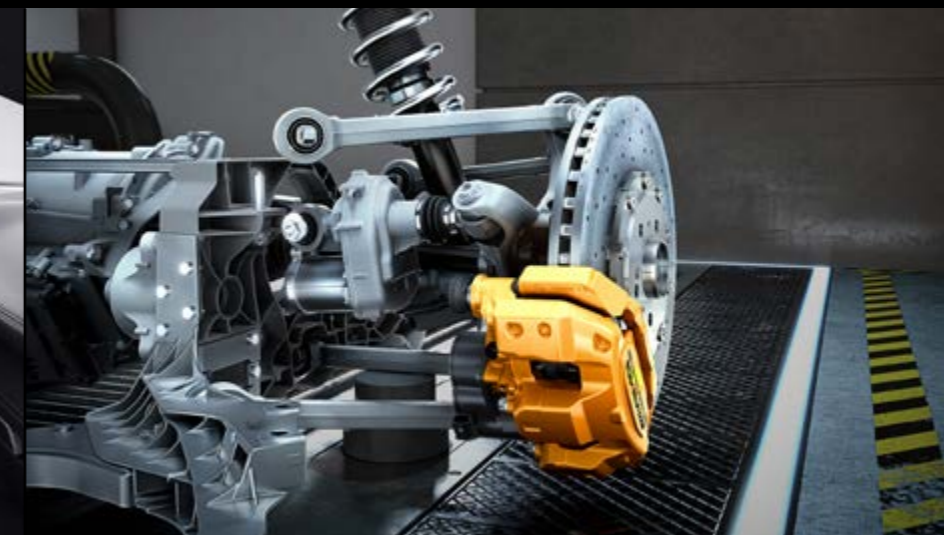
201 - Asse sterzante posteriore
